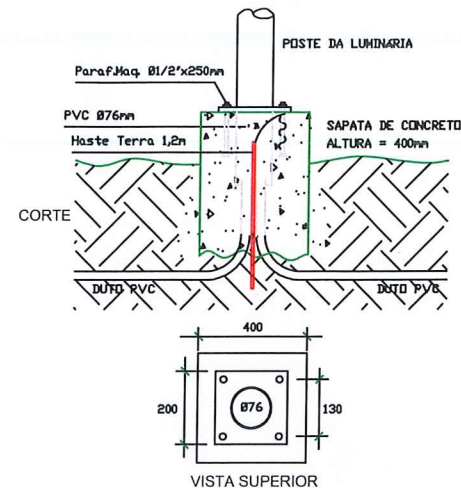
DETALHE DA FIXAÇÃO DOS POSTES DE 3000mm Ø76mm SEM ESCALA
