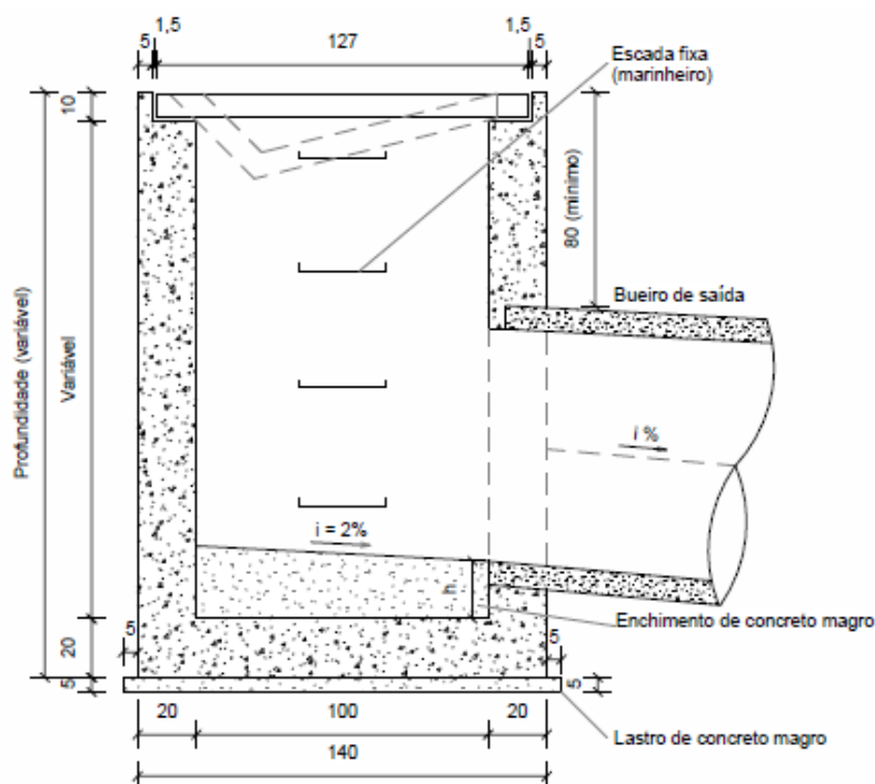
Corte A-A' Sem escala
