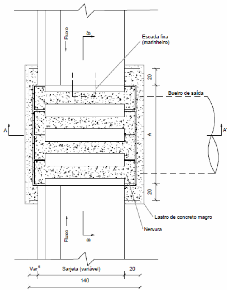
Planta Sem escala
