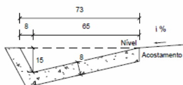
Seção transversal Escala 1 : 20
