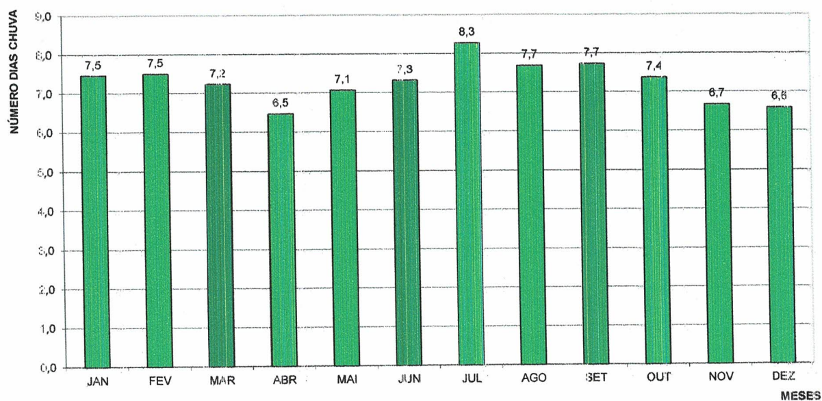
Figura 3 - Histograma da média histórica das chuvas mensais.
