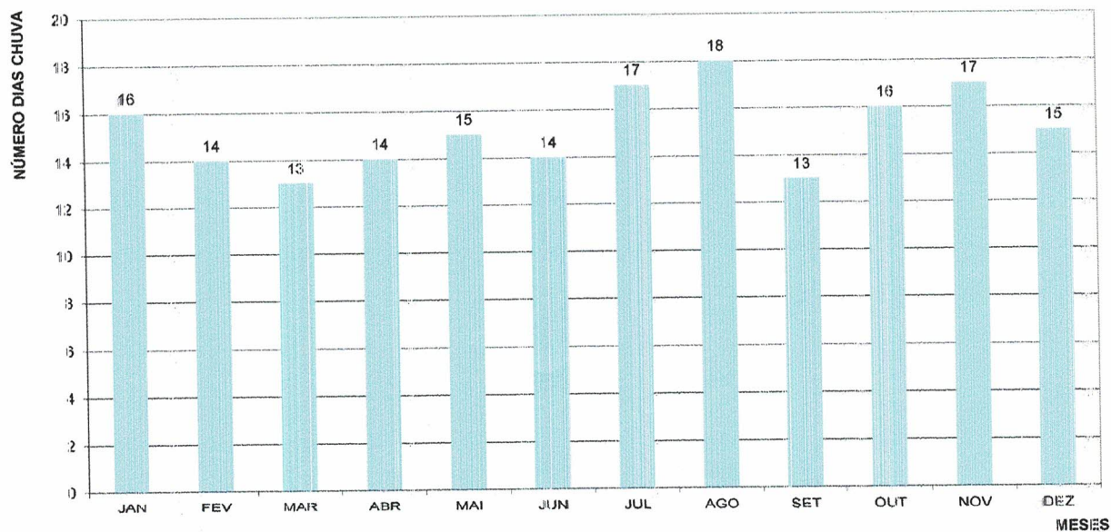
Figura 4 - Histograma da máxima histórica dos dias de chuvas mensais.
