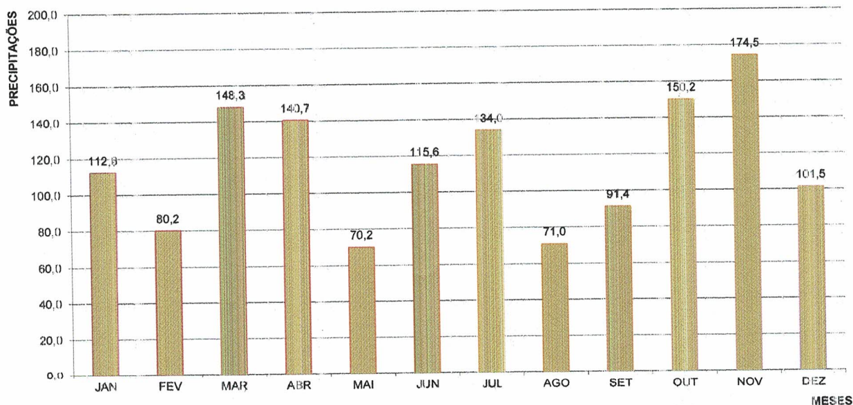
Figura 2 - Histograma da máxima histórica das precipitações máximas mensais.
