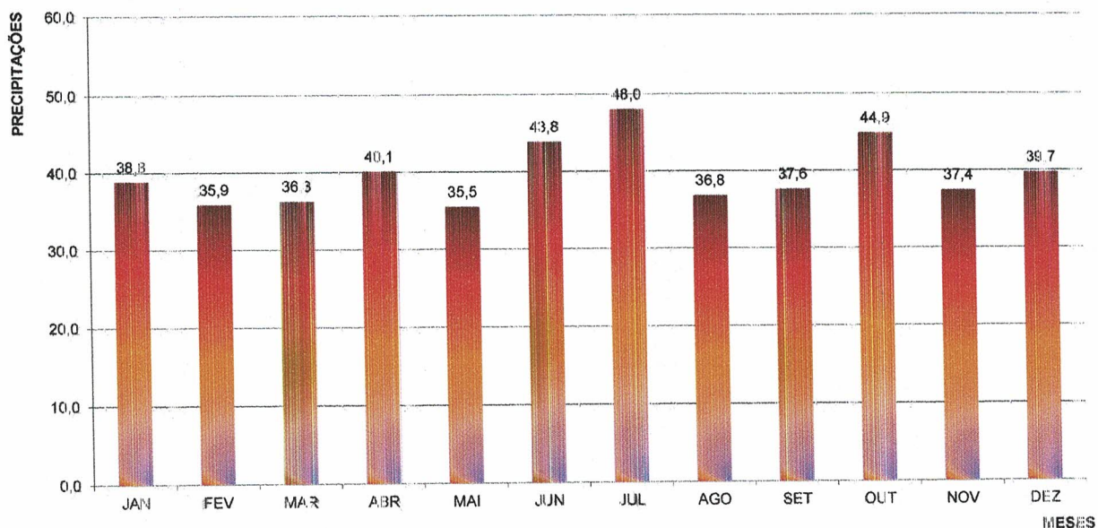
Figura 1 - Histograma da média histórica das precipitações máximas mensais.
