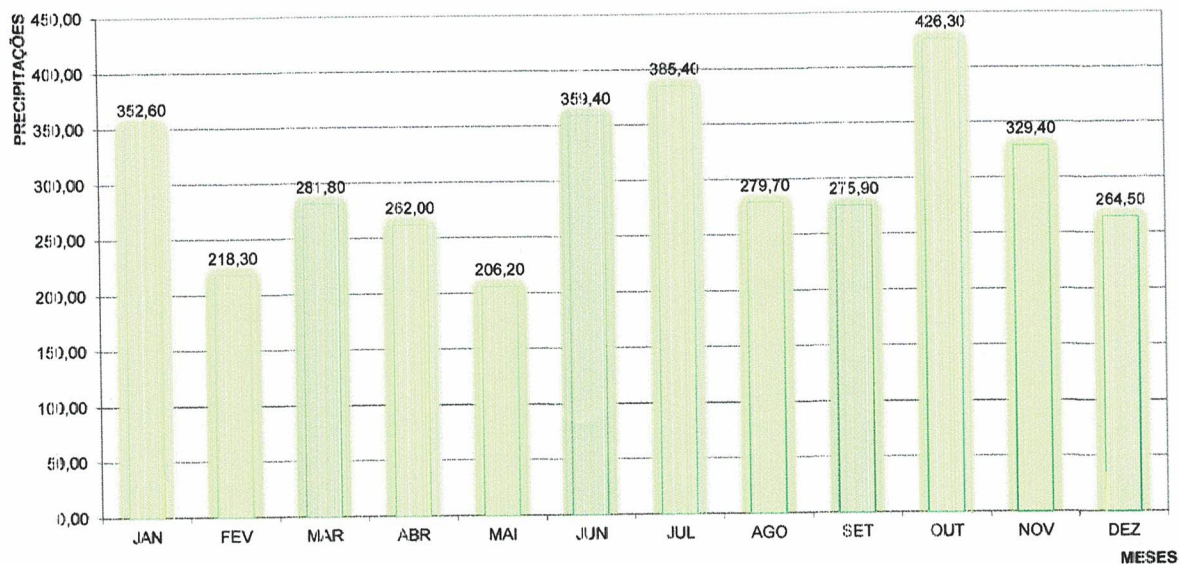
Figura 6 - Histograma da máxima histórica das precipitações totais mensais.
