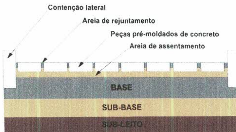
FOTO: 01 - Esquema da Estrutura do Pavimento.
