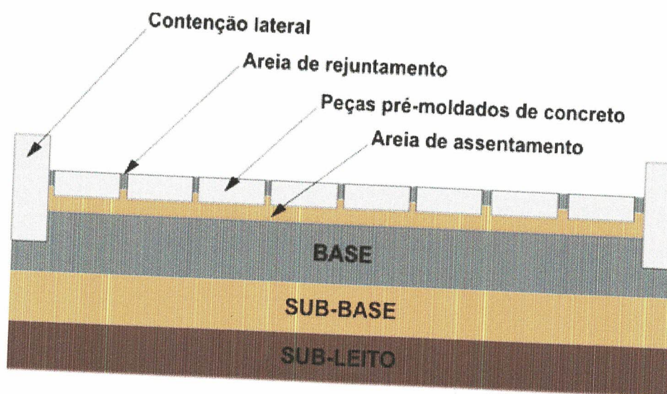
FOTO: 01 - Esquema da Estrutura do Pavimento.
