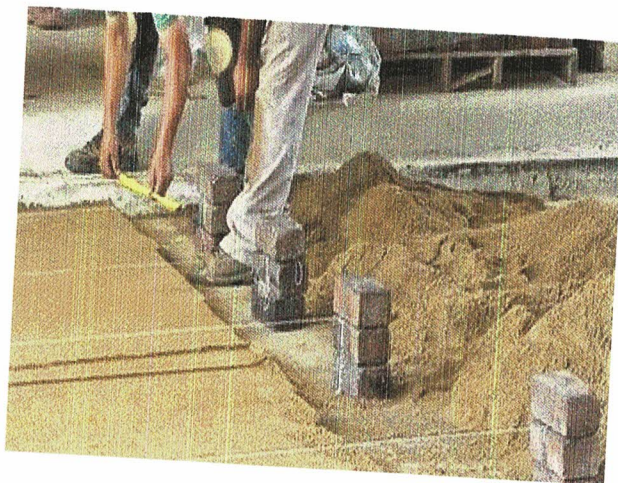
FOTO: 03, Colchão de Areia para assentamento PAVs.
