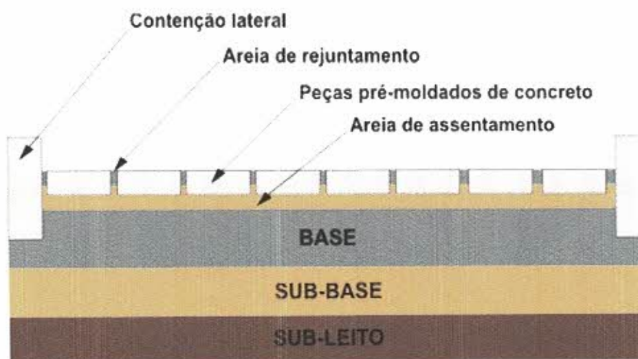
FOTO: 5 - Esquema da Estrutura do Pavimento.
